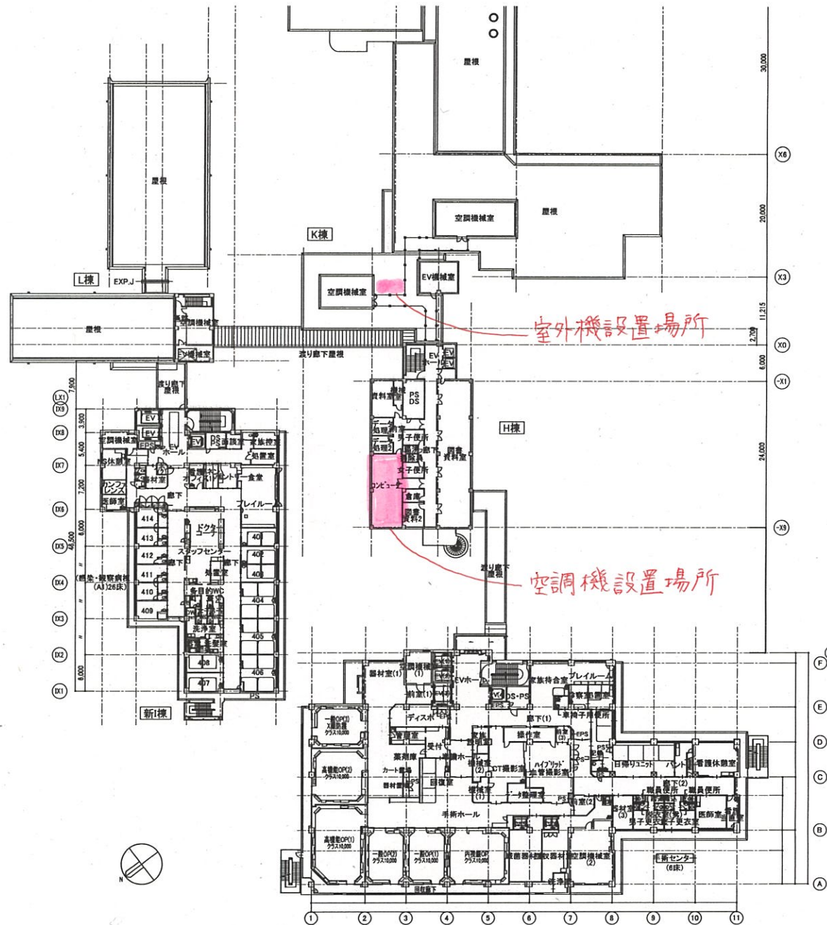
静岡県立こども病院 4階平面図 2015.8.25 1/600
