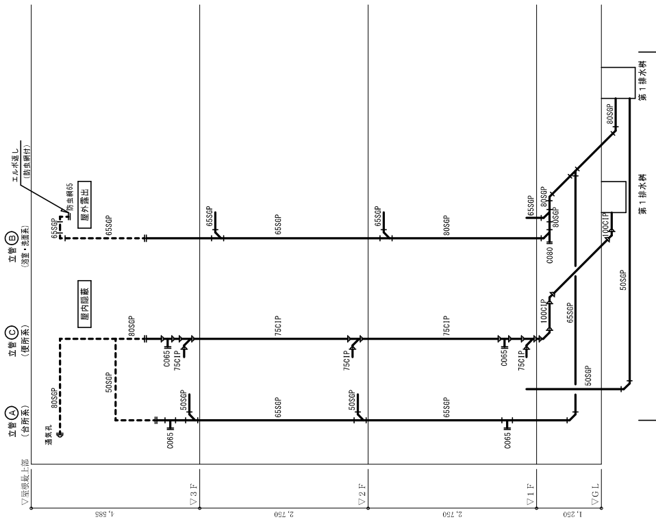
配管系統図 N.S. ※上図は排水系1系統分を示す。
