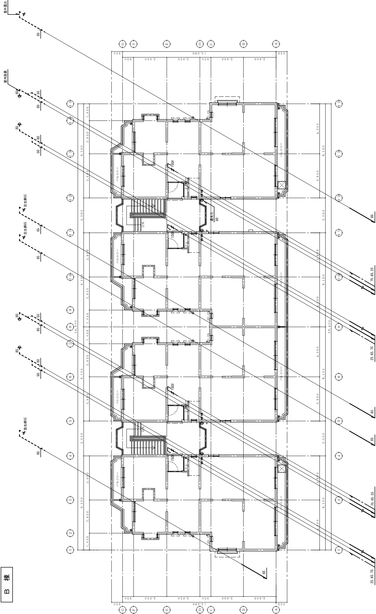
3階 平面図 S:1/100 ※給水管は参考
