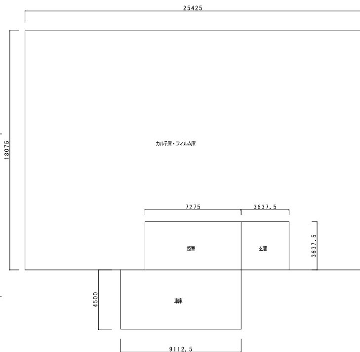
居室床面積算定図 A1:S=1/100, A3:S=1/200
