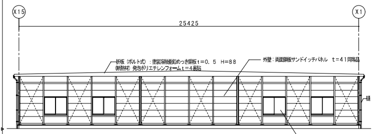
Y11通り立面図 A1:S=1/100, A3:S=1/200
