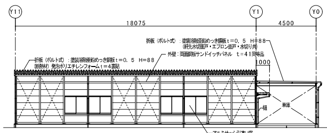
X1通り立面図 A1:S=1/100, A3:S=1/200
