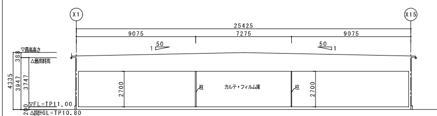
A-A 断面図 A1: S=1/100, A3: S=1/200
