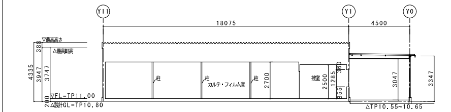
B-B 断面図 A1: S=1/100, A3: S=1/200
