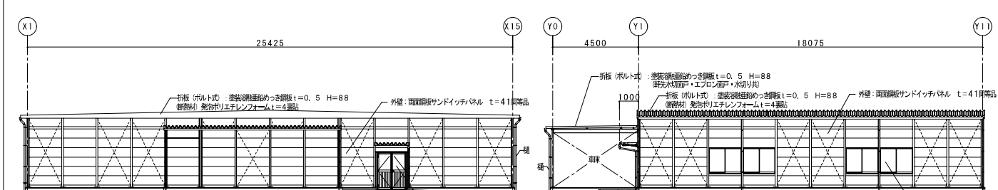
Y0通り立面図 A1:S=1/100, A3:S=1/200
